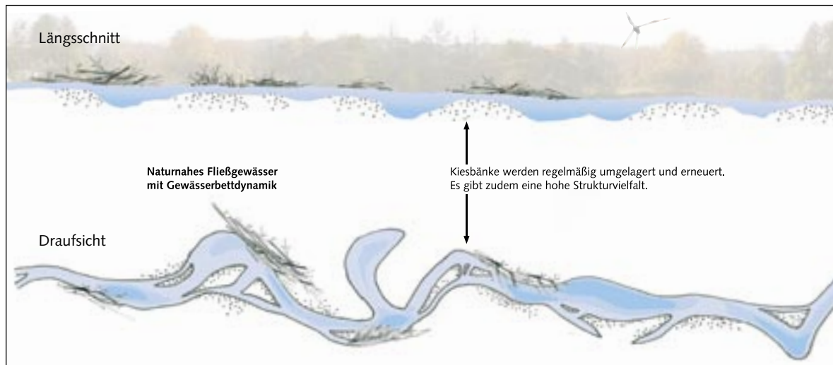
Schema eines naturnahen dynamischen Fließgewässers. Durch natürlichen Geschiebetransport entstehen Kieslaichplätze von selbst.
